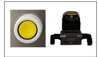
07 PULSADOR DE LAVADO DISOLVENTE LIMPIO WASHING PUSH BUTTON CLEAN SOLVENT
